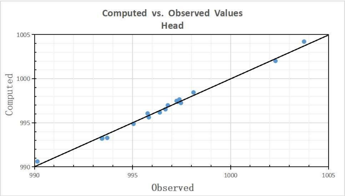
图 6.2-7 数值模型计算、观测水位对比图
