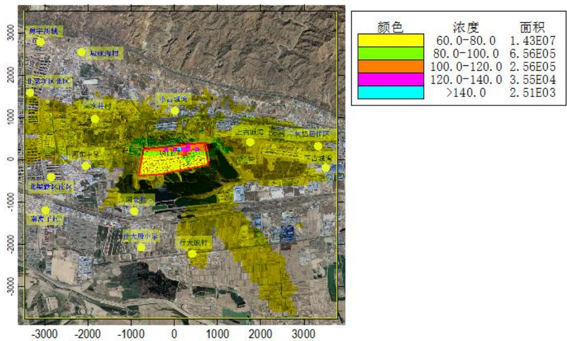
图 6.1-35 叠加后 TSP24 小时平均浓度等值线分布图（单位：μg/m³）
