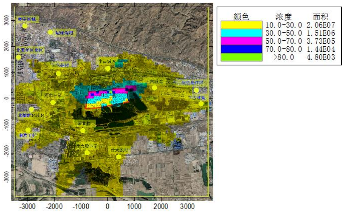
图 6.1-17 TSP24 小时平均质量浓度贡献值分布图（单位： \mu\text{g}/\text{m}^3 ）
