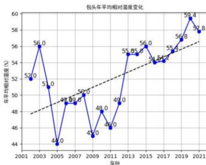
图 6.1-10 包头近 20 年平均相对湿度（纵轴为百分比，虚线为趋势线）
