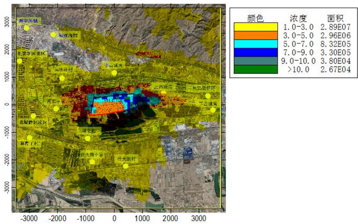
图 6.1-19 PM 10 24 小时平均质量浓度贡献值分布图（单位：μg/m 3 ）
