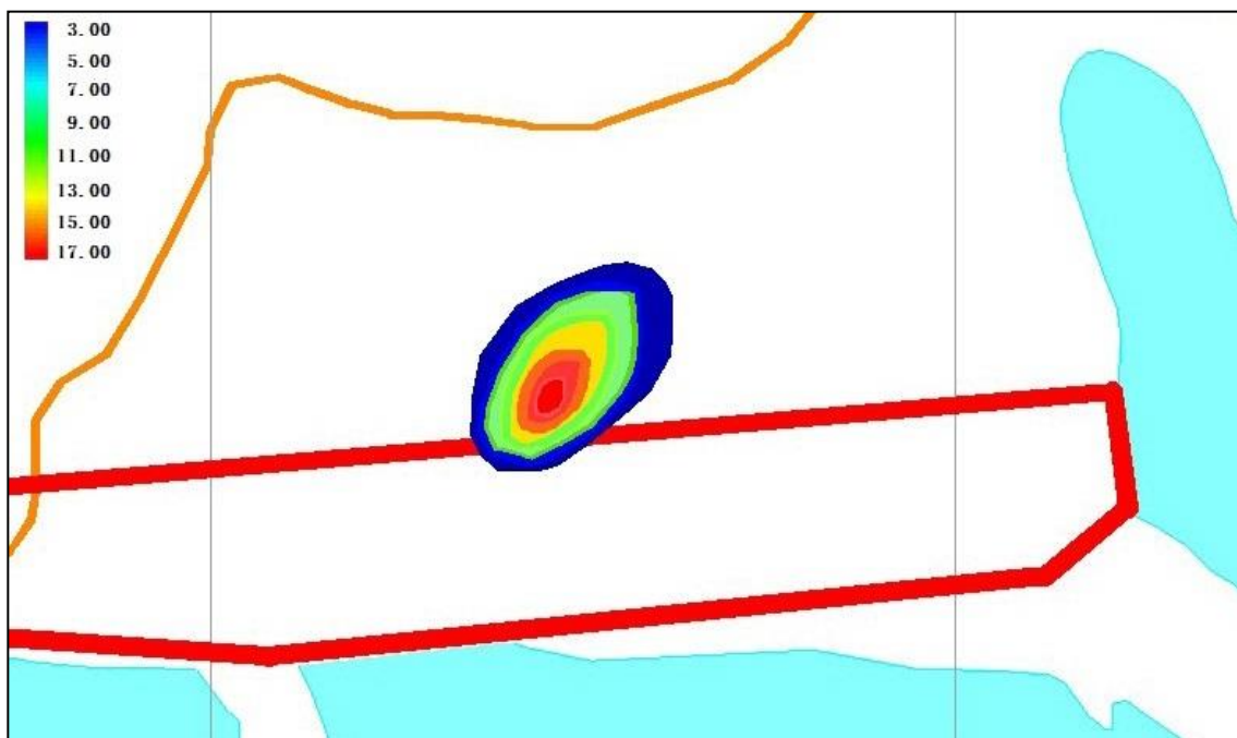
图 6.2-10 COD 1250d 污染晕运移图
