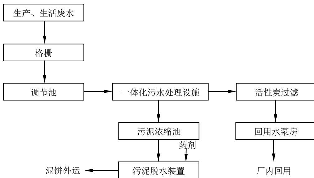
图 6.3-1 包铝四期污水处理站工艺流程图
