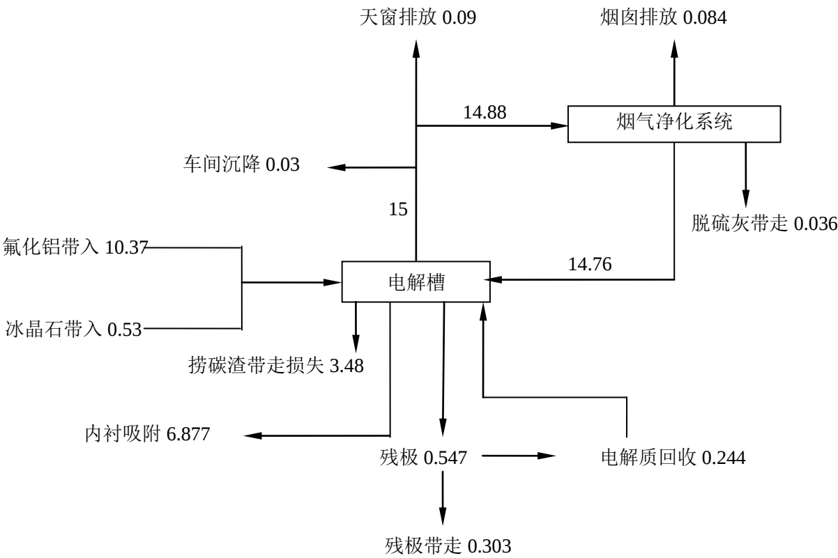
图 4.2-2 华云三期氟平衡图 单位：kg/t-Al
