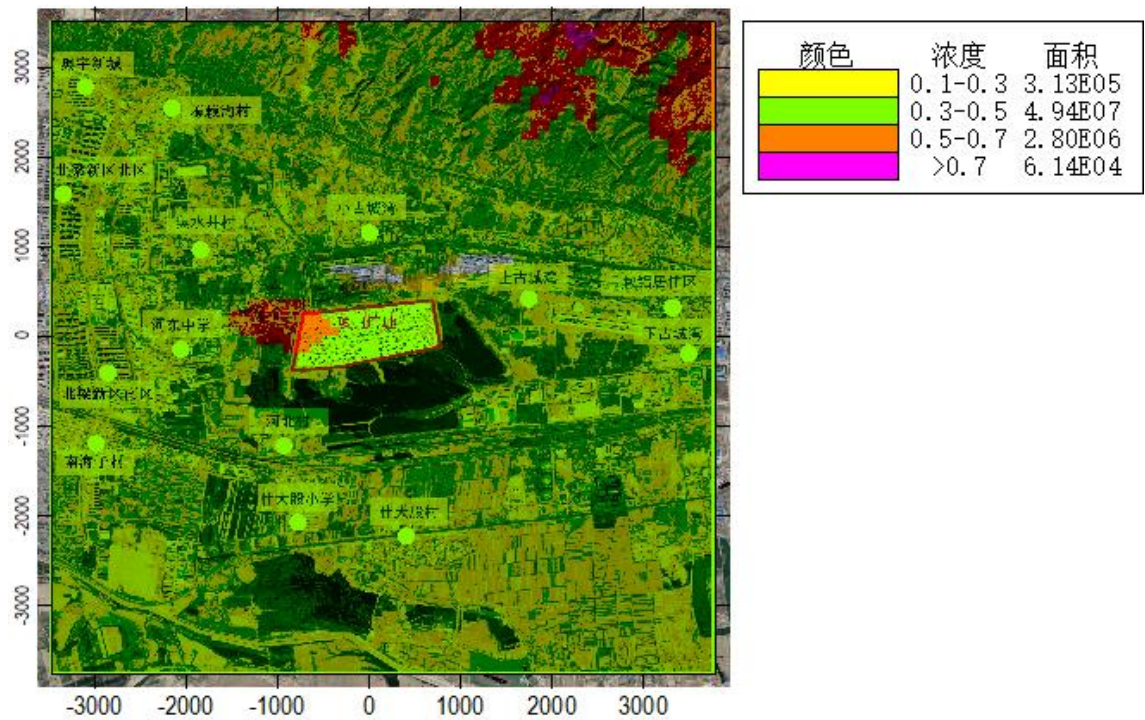
图 6.1-34 叠加后氟化物 24 小时平均浓度等值线分布图（单位：μg/m 3 ）
