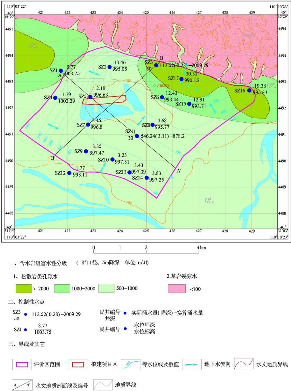
图 6.2-1 评价区水文地质图
