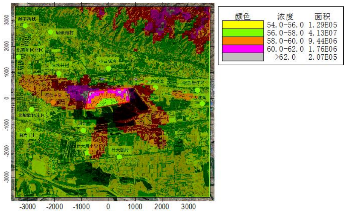
图 6.1-31 叠加后 PM 2.5 24 平均浓度等值线分布图（单位：μg/m 3 ）
