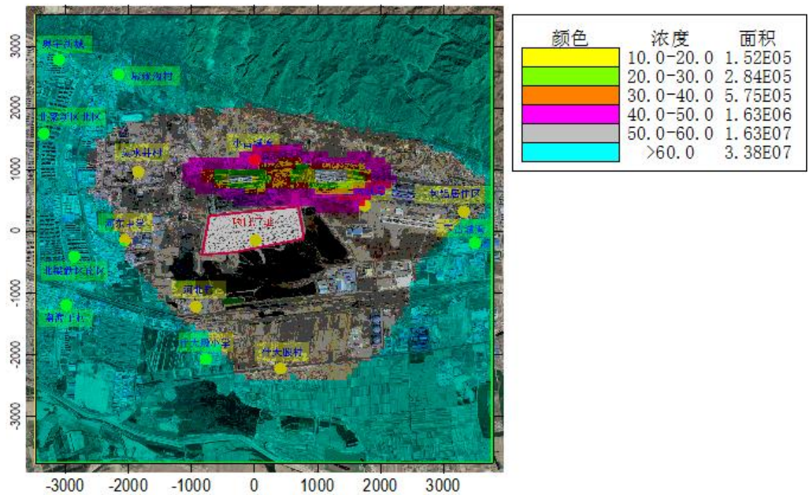
图 6.1-30 叠加后 PM 10 年平均浓度等值线分布图（单位：μg/m 3 ）
