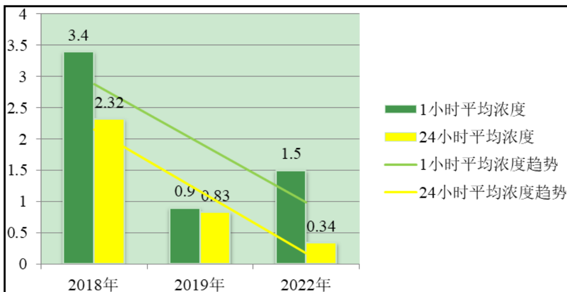
图 5.4-8 氟化物短期浓度趋势图
