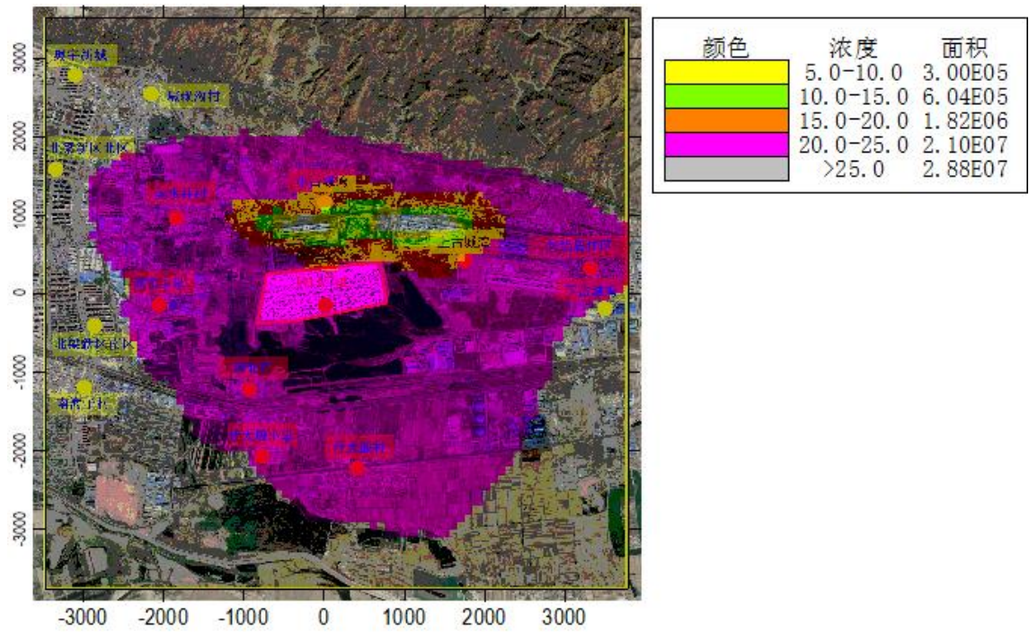
图 6.1-32 叠加后 PM 2.5 年平均浓度等值线分布图（单位：μg/m 3 ）
