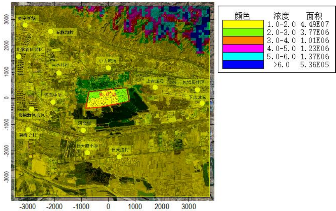
图 6.1-33 叠加后氟化物 1 小时平均浓度等值线分布图（单位：μg/m 3 ）
