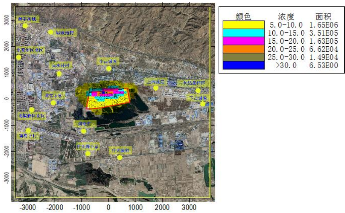
图 6.1-18 TSP 年均质量浓度贡献值分布图（单位： \mu\text{g}/\text{m}^3 ）
