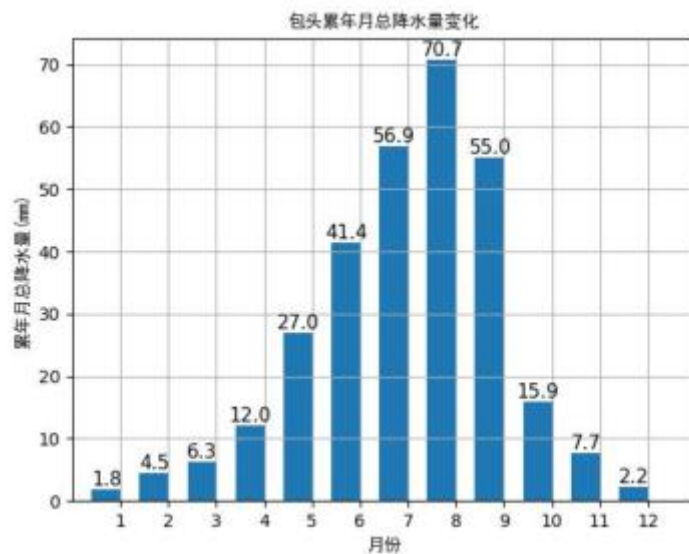
图 6.1-5 包头月平均降水量 (单位: 毫米)
