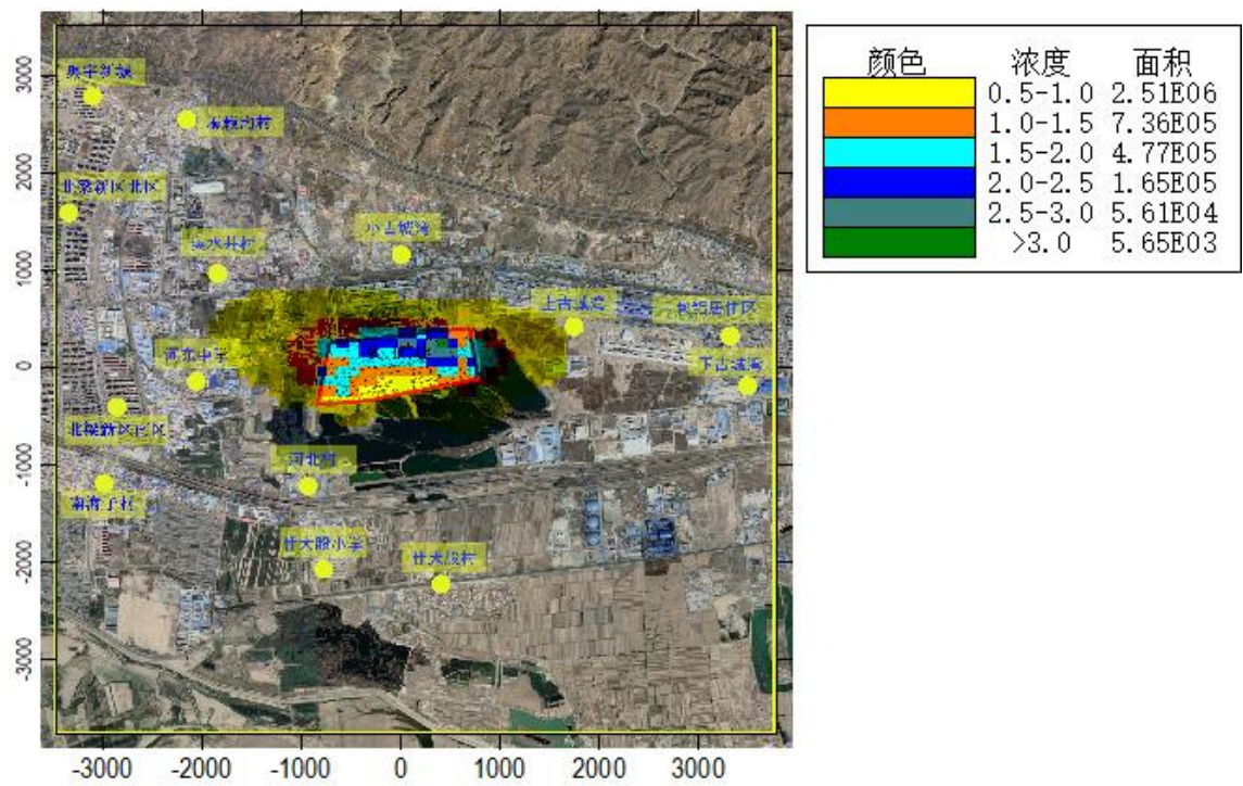
图 6.1-20 PM 10 年平均质量浓度贡献值分布图（单位：μg/m 3 ）
