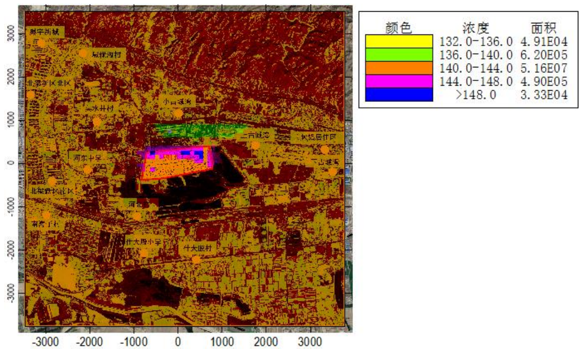
图 6.1-29 叠加后 PM 10 24 小时平均浓度等值线分布图（单位：μg/m 3 ）
