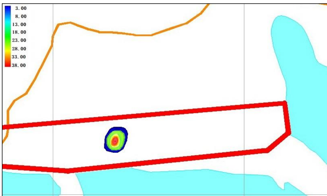
图 6.2-9 COD 200d 污染晕运移图
